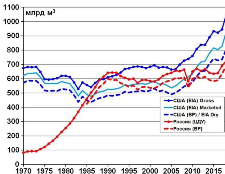
Рис.5.2. Сопоставление объемов добычи газа в США и России по данным различных источников (EIA, BP, ЦДУ ТЭК) [29]
