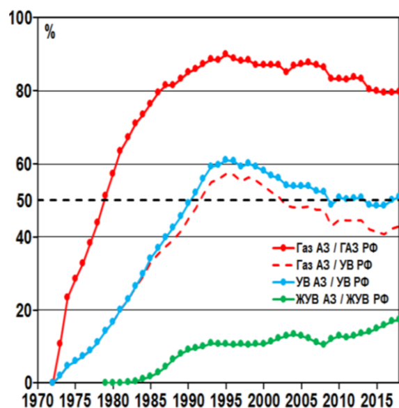
Рис. 5.11. Доли добычи углеводородов в АЗРФ в общем объеме добычи России
