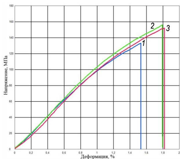
Рис. 4. Типичные деформационные кривые нанокompозита на изгиб при полимеризации при температуре: 24 °C (1), 45 °C (2) и 70 °C (3) [7]
