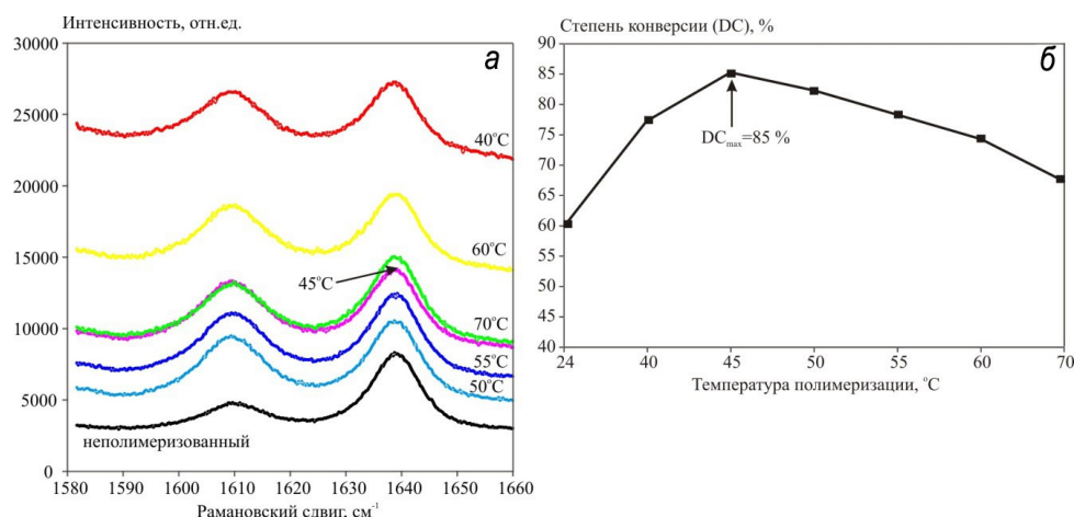
Рис. 2. Рамановские спектры в области 1580\text{--}1660\text{ см}^{-1} (а) и зависимость степени конверсии метакрилатной матрицы композита Filtek Ultimate от температуры полимеризации (б), оцененная по данным рамановской спектроскопии [1]
