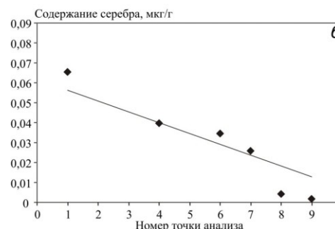
Рис. 5. СЭМ-изображение дентина с точками, в которых проводилась лазерная абляция (а), содержание Ag в дентине после обработки стоматологическим протравочным гелем Etchmaster Ag™ (б) [1]
