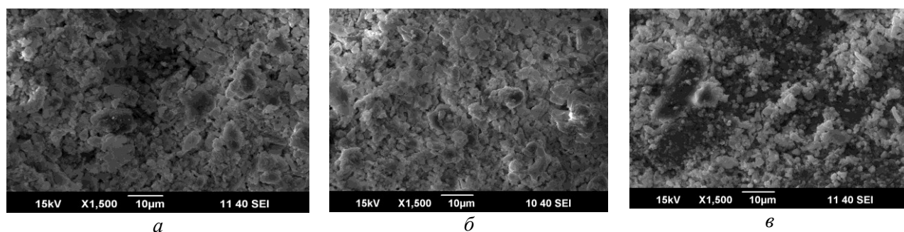
Рис. 3. Изображения фрагментов композитного материала, полимеризованного при температуре: 24 °C (а), 45 °C (б) и 70 °C (в) [2]
