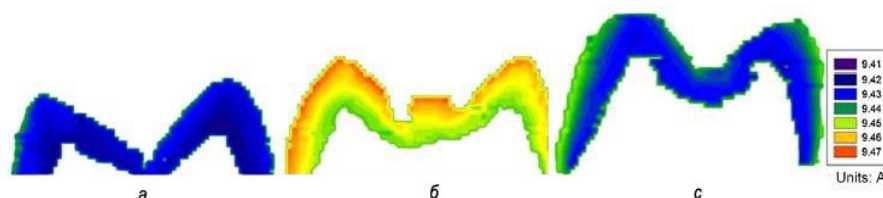
Рис. 6. Карты пространственного распределения параметра кристаллической решетки a (Å) гидроксиапатита эмали зуба трех различных стадий зрелости: а — ранней (1,5 года); б — средней (2,5 года); в — полной (10 лет) [11]
