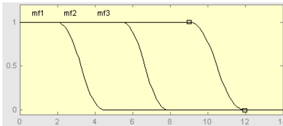
Рис. 3. Терм-множество выходного параметра «Напряжение задания по скорости»
