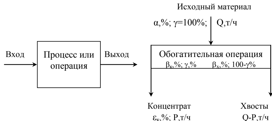
Рис. 1. Входные и выходные параметры разделительного процесса \alpha - содержание полезного компонента в питании; \beta_k - содержание полезного компонента в концентрате; \beta_x - содержание компонента в хвостах; \epsilon_k - извлечение полезного компонента в концентрат
