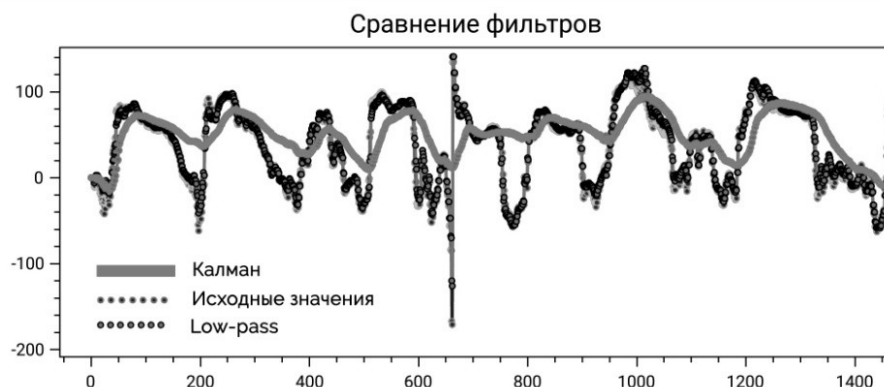
Рис. 3. Сравнение исходных данных датчиков с данными, полученными в результате применения фильтров нижних частот и Калмана
