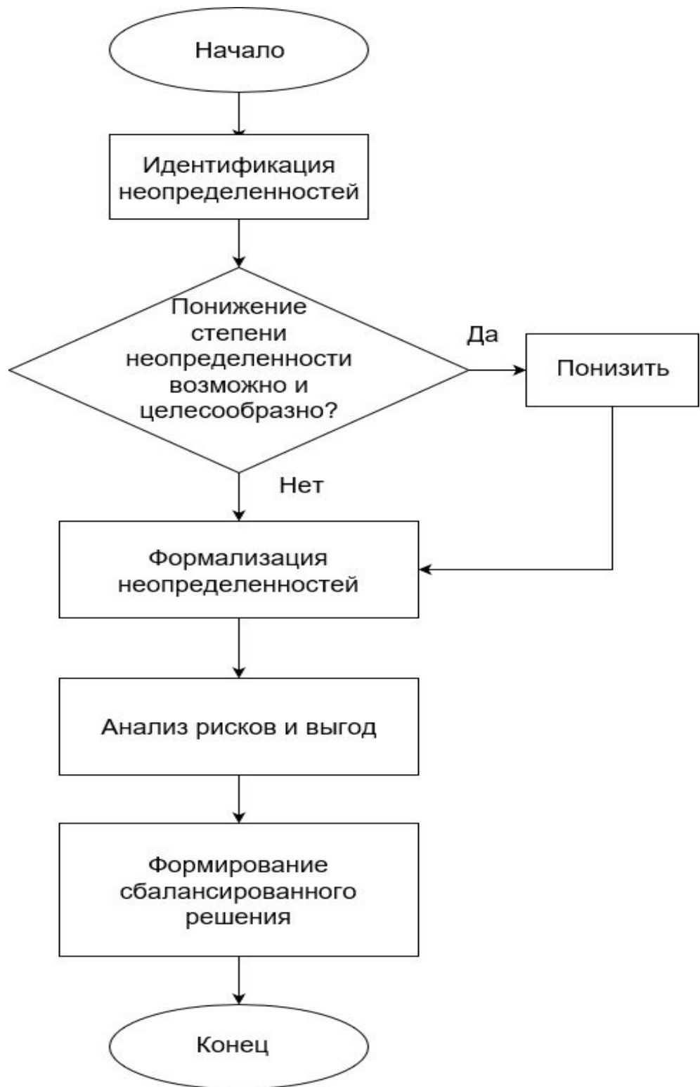
Алгоритм управления безопасностью с учётом неопределённостей
