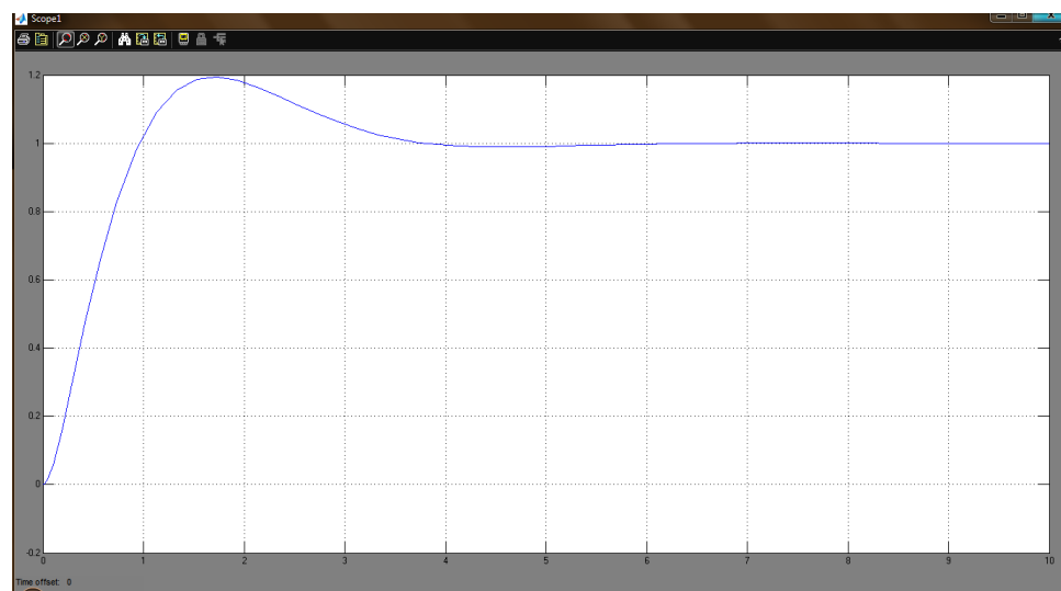
Рис. 7. График изменения производительности конусной дробилки при пуске (нечёткий регулятор)
