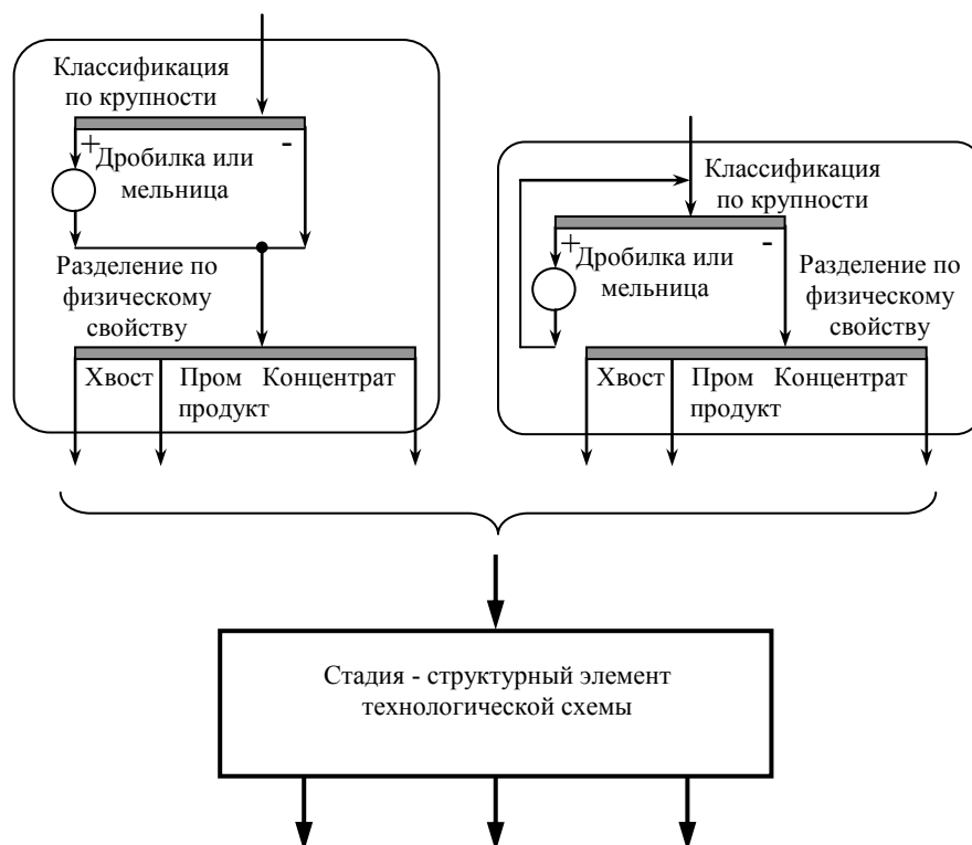
Рис. 2. Структурный элемент декомпозиции технологической схемы
