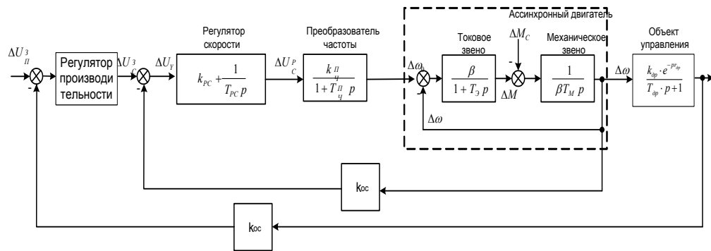
Рис. 1. Структурная схема системы регулирования производительности конусной дробилки
