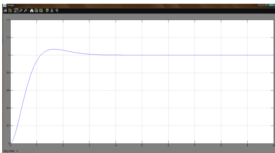
Рис. 5. График изменения производительности конусной дробилки при пуске (ПИИ-регулятор)
