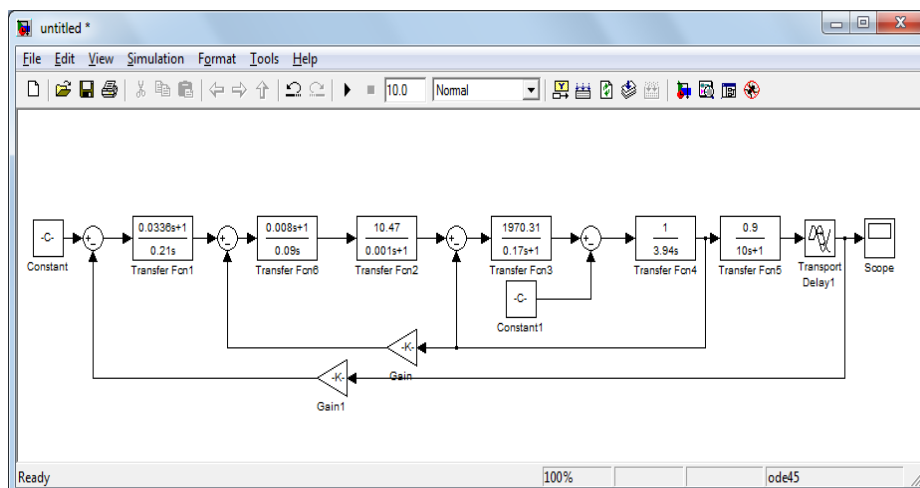
Рис. 4. Математическая модель системы автоматического регулирования производительности конусной дробилки (ПИИ-регулятор)
