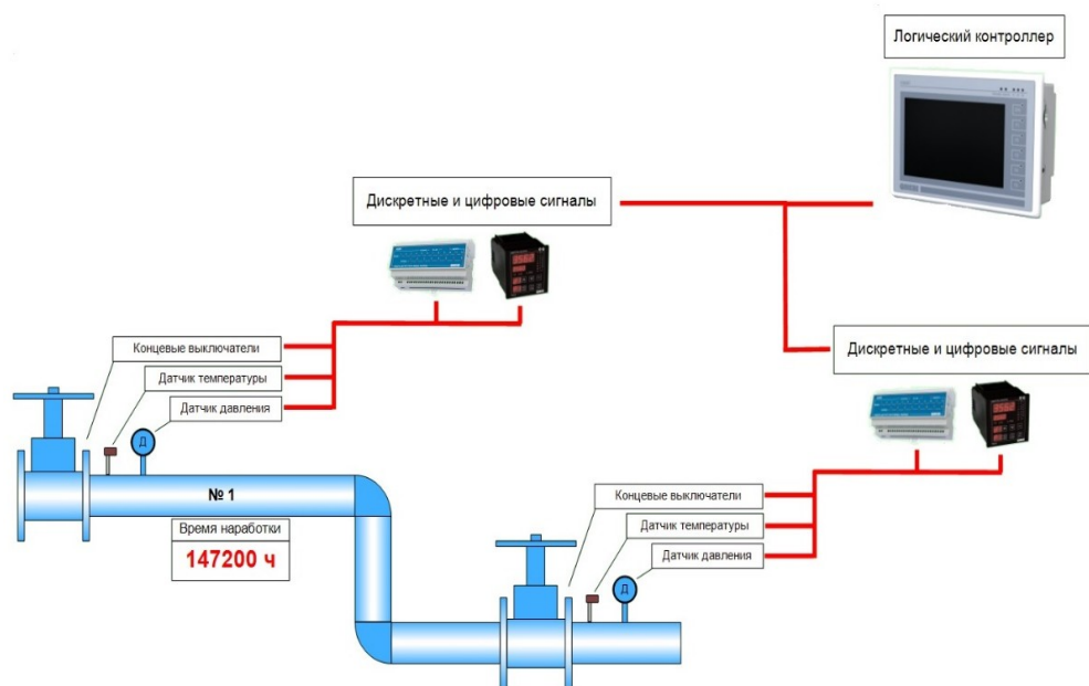
Рис. 2. Структурная схема системы автоматического учета наработки элементов паропровода с отображением рабочих параметров в режиме реального времени
