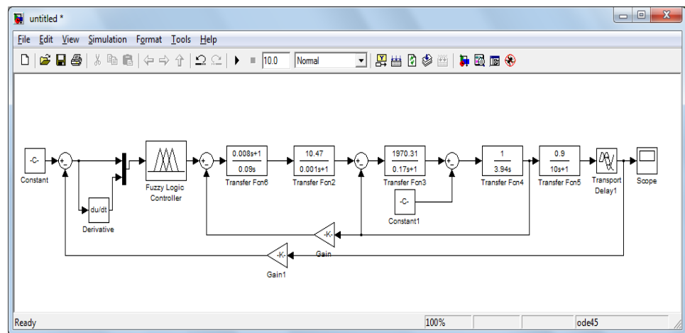
Рис. 6. Математическая модель системы автоматического регулирования производительности конусной дробилки (нечёткий регулятор)
