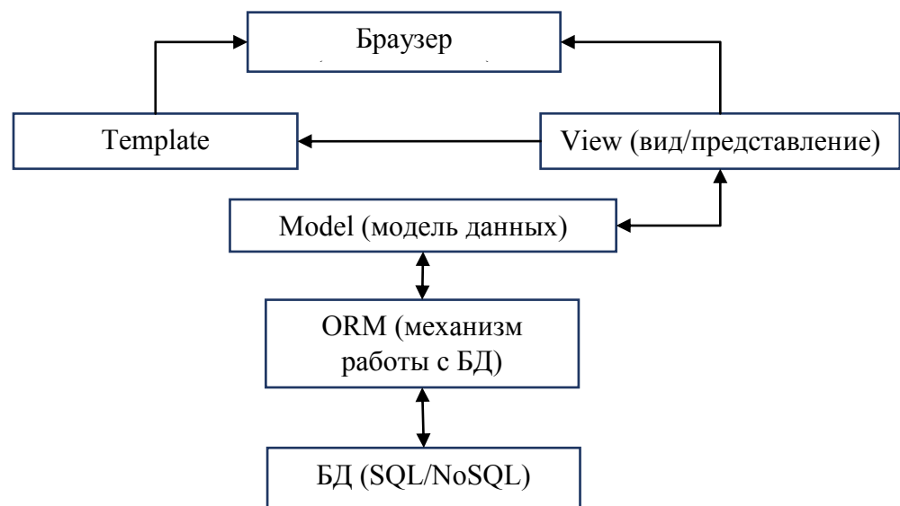
Архитектура MTV
