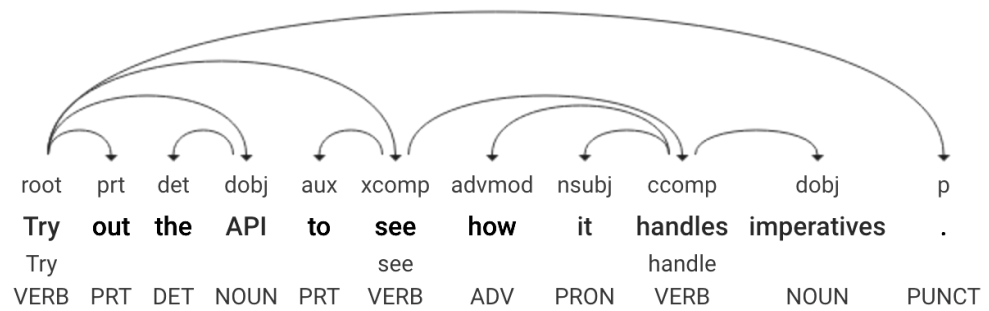
Рис. 2. Пример синтаксического разбора предложения
