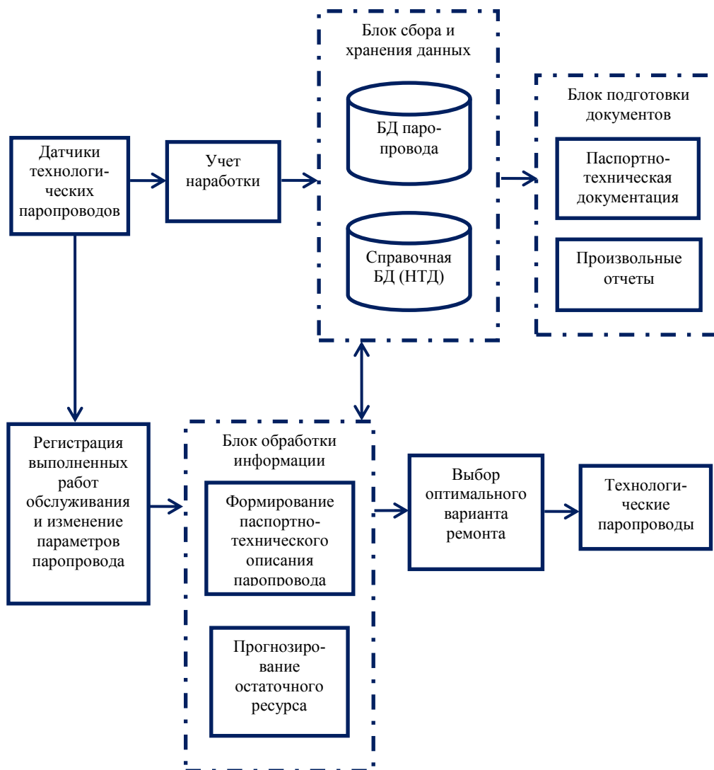
Рис. 3. Структурная схема системы мониторинга и прогнозирования состояния паропроводов
