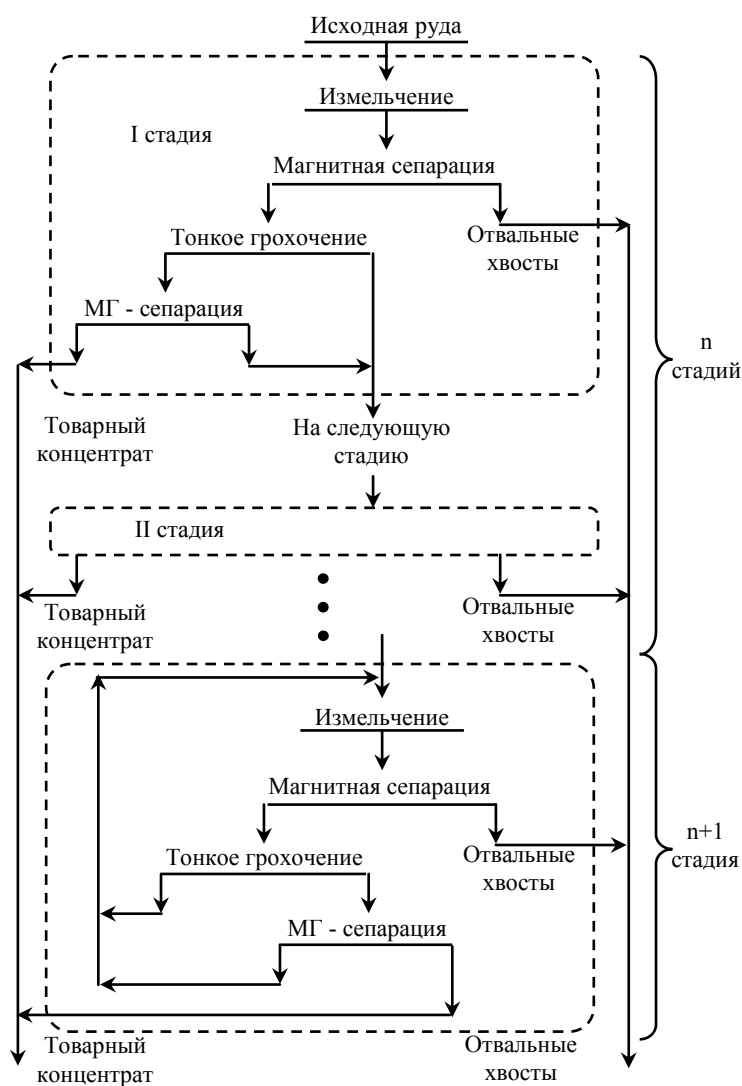
Рис. 3. Перспективная технологическая схема переработки железистых кварцитов
