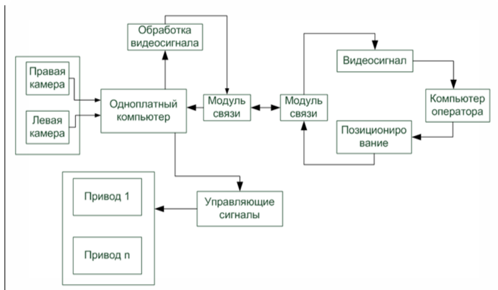
Рис. 1. Архитектура программно-аппаратного комплекса
