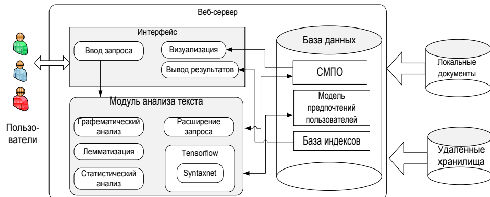
Рис. 3. Веб-сервис семантического индексирования
