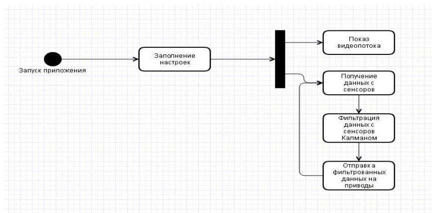
Рис. 4. Диаграмма Activity
