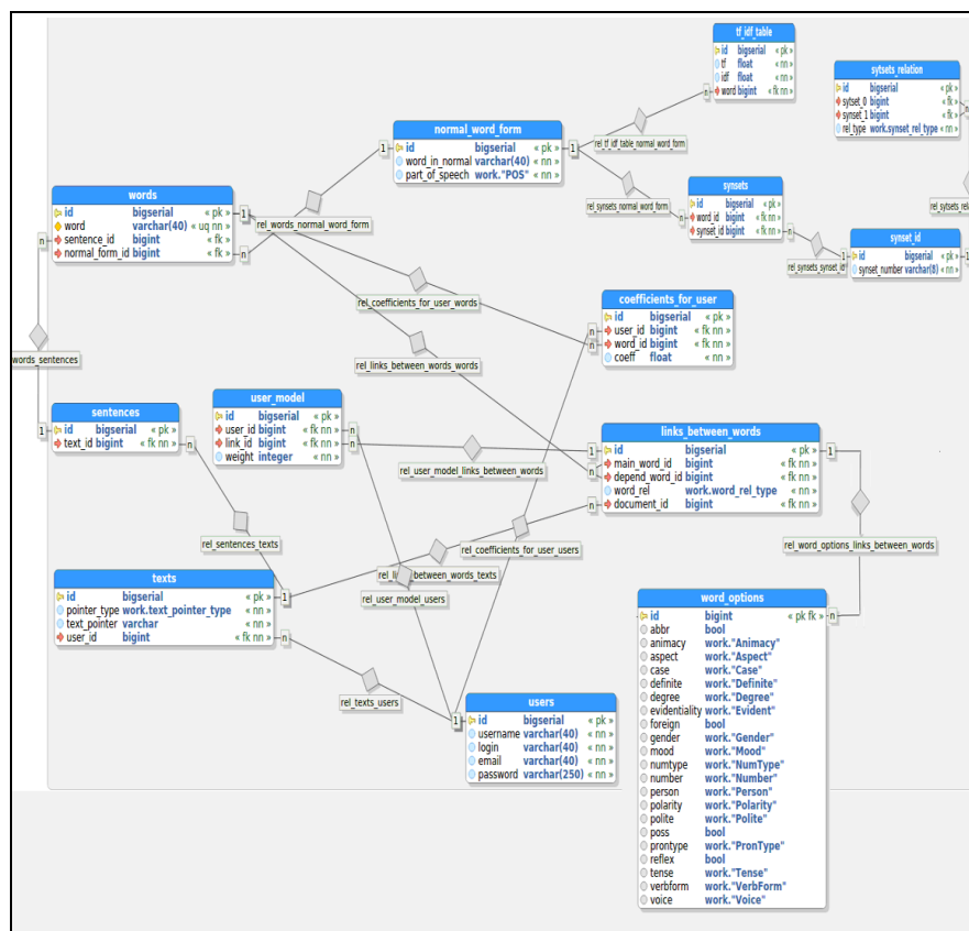
Рис. 4. Схема данных для хранения семантической модели предметной области
