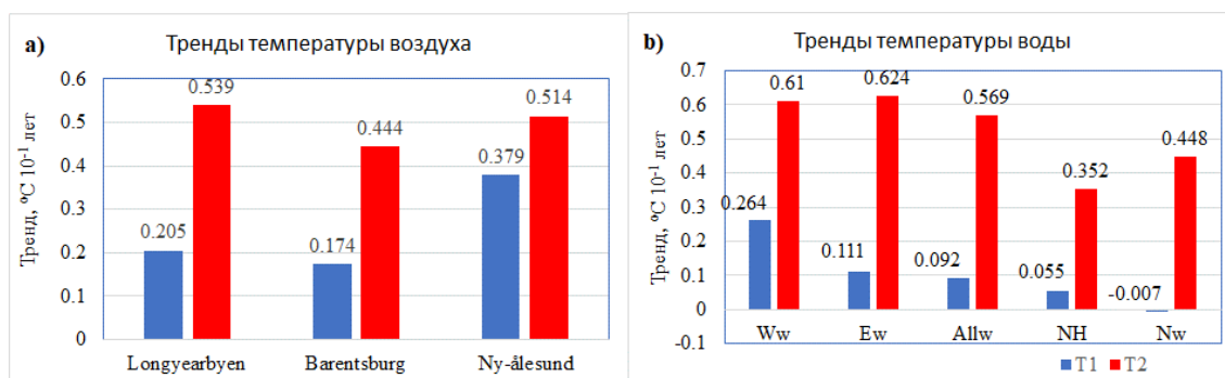
Рис. 2. Линейные тренды T1 и T2 на метеостанциях архипелага Шпицберген (а) и на акваториях, омывающих архипелаг (б)
